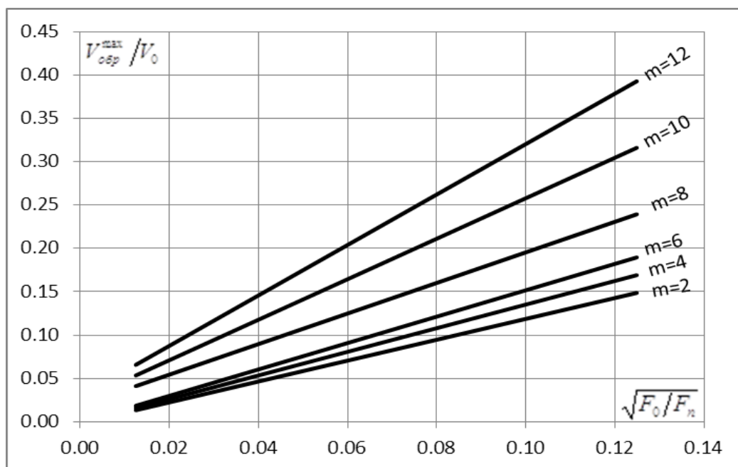
Рисунок Ж.2 – Зависимость максимальной скорости в обратном потоке от параметра \sqrt{F_0 / F_{\Pi}} стеснения и кинематического коэффициента m ВР
