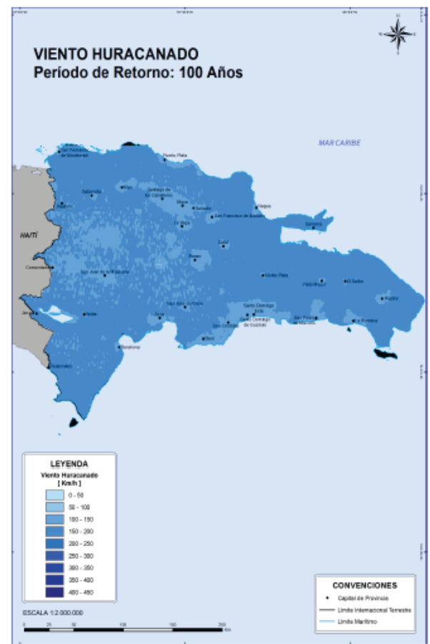
Figura 7: Vientos huracanado por periodos de retorno de 100 años (BID 2012)
